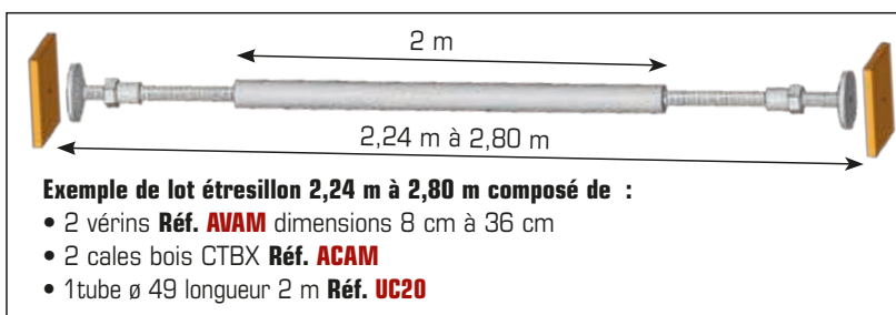
Amarrage en fenêtre avec : lot étreillon + colliers à clavettes ou raccords à boulons + tubes + cales bois.
