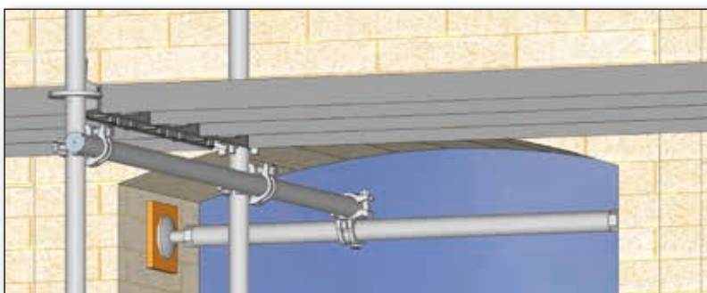
Amarrage en fenêtre avec : lot étreillon + colliers à clavettes ou raccords à boulons + tubes + cales bois.
